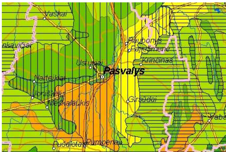
3-11 pav. Lietuvos kraštovaizdžio geocheminės toposistemos (Šaltinis: http://www.am.lt/VI/files/File/kraštovaizdis/leidiniai/Geochtopo.jpg )
